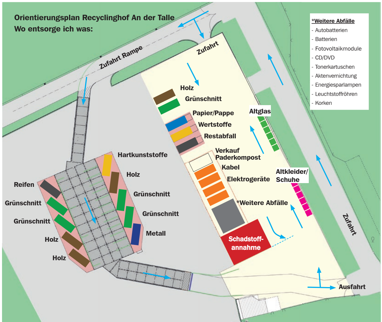
Abbildung 3: Flächenaufteilung und Containeranordnung auf dem Recyclinghof
